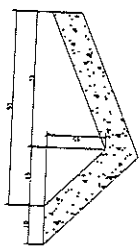
SARJETA TIPO 40/15 ESC: 1/5
